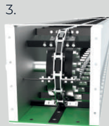
1. Batea; 2. Caño cuadrado; 3. Piso de redler; 4. Caño redondo; 5. Cabezal noria
